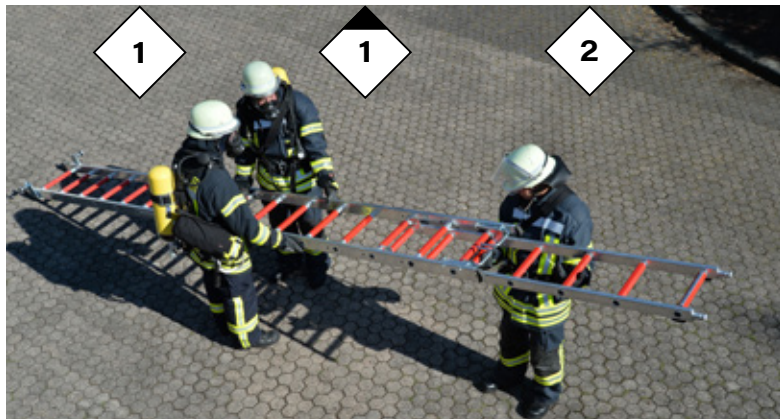
Abb. 34: Aufstecken des Aufsteckteils
