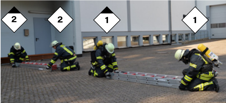
Abb. 38: Vorbereiten der Multifunktionsleitern
